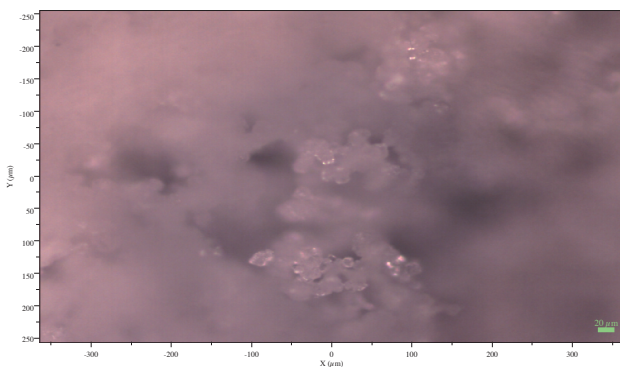
炭酸カルシウムの結晶の顕微鏡写真
