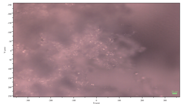
シュウ酸カルシウムの結晶の顕微鏡写真
